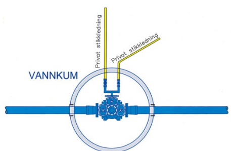
Figur 2: Illustrasjonen viser hva som er kommunal og privat ledning i en vannkum.
