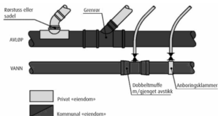
Figur 1: Illustrasjonen viser hvilke rørdeler som er privat og kommunal eiendom.
